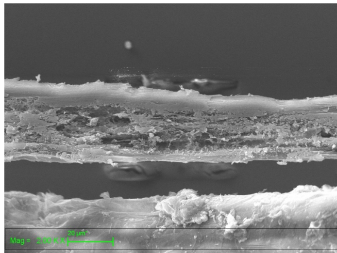
Рисунок 5. Микрофотографии волокон шерсти, сделанные с помощью СЭМ (текстильные образцы из Усть-Войкарского городища)
