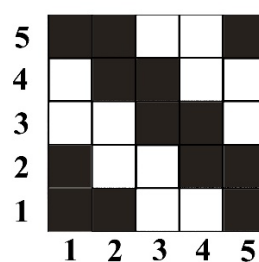
Б Саржевое переплетение (саржа 2/2)
